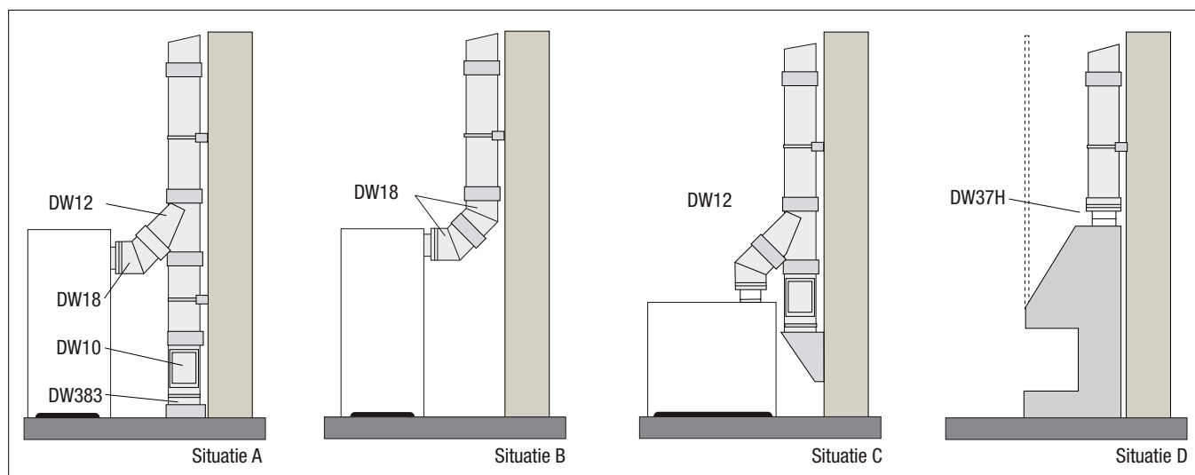
Figuur 12 - Montage stormkraag
