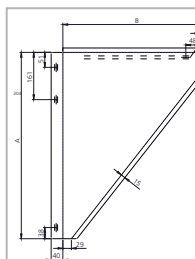
Konsoleplaten verstelbaar 250 - 360mm / ADWECO49
