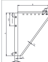
Konsoleplaten verstelbaar 150 - 250mm / ADWECO02
