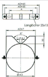
Muurbeugel 50 mm / ADWECO87H
