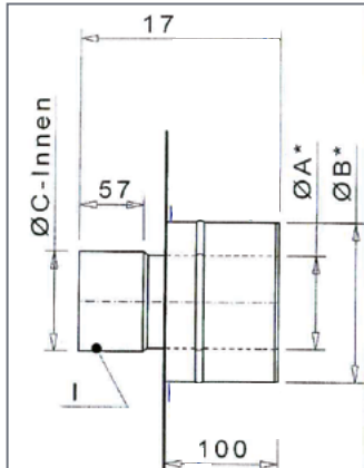
Verloop FLEX/TWIN / HTWIN465
