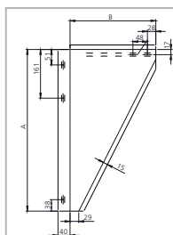
Konsoleplaten verstelbaar 50 - 150mm / DWECO01
